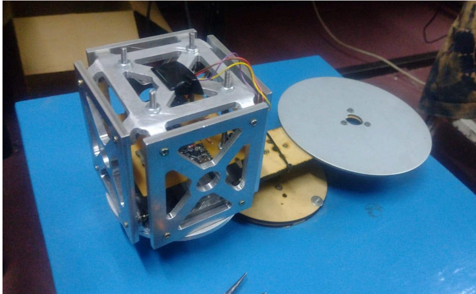
Figura 23: CubeSAT montado en el equipo confeccionado para el ensayo de aceleración cuasiestática.
